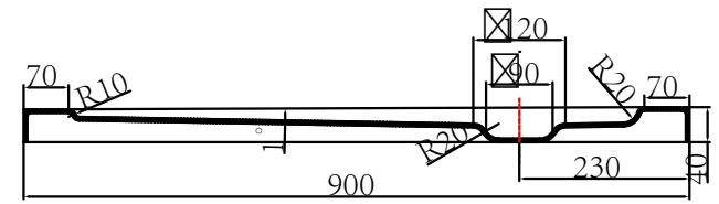
Scetion A-A
